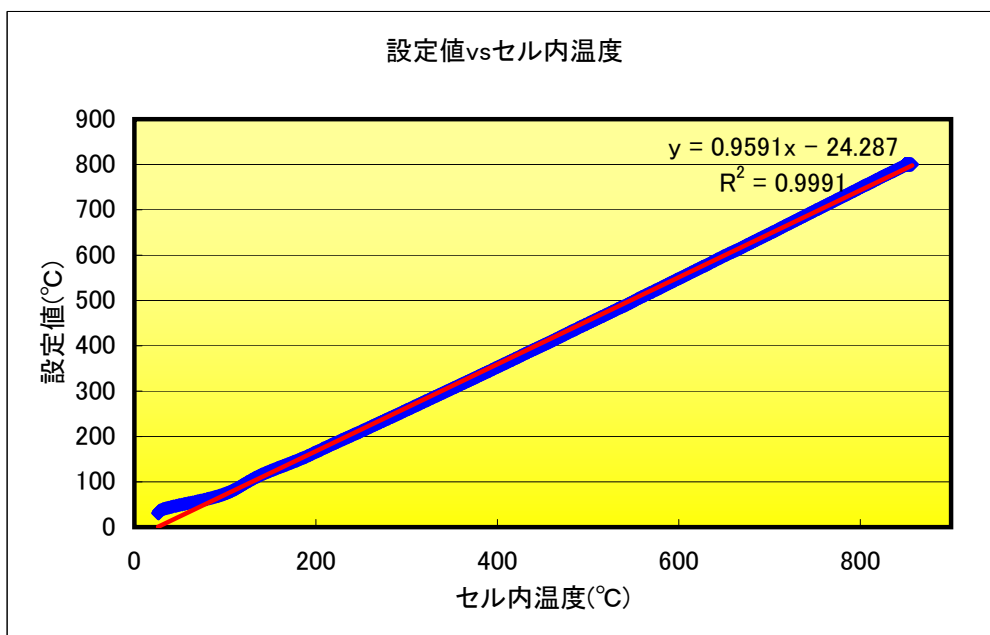
図1 設定値 vs セル内温度
