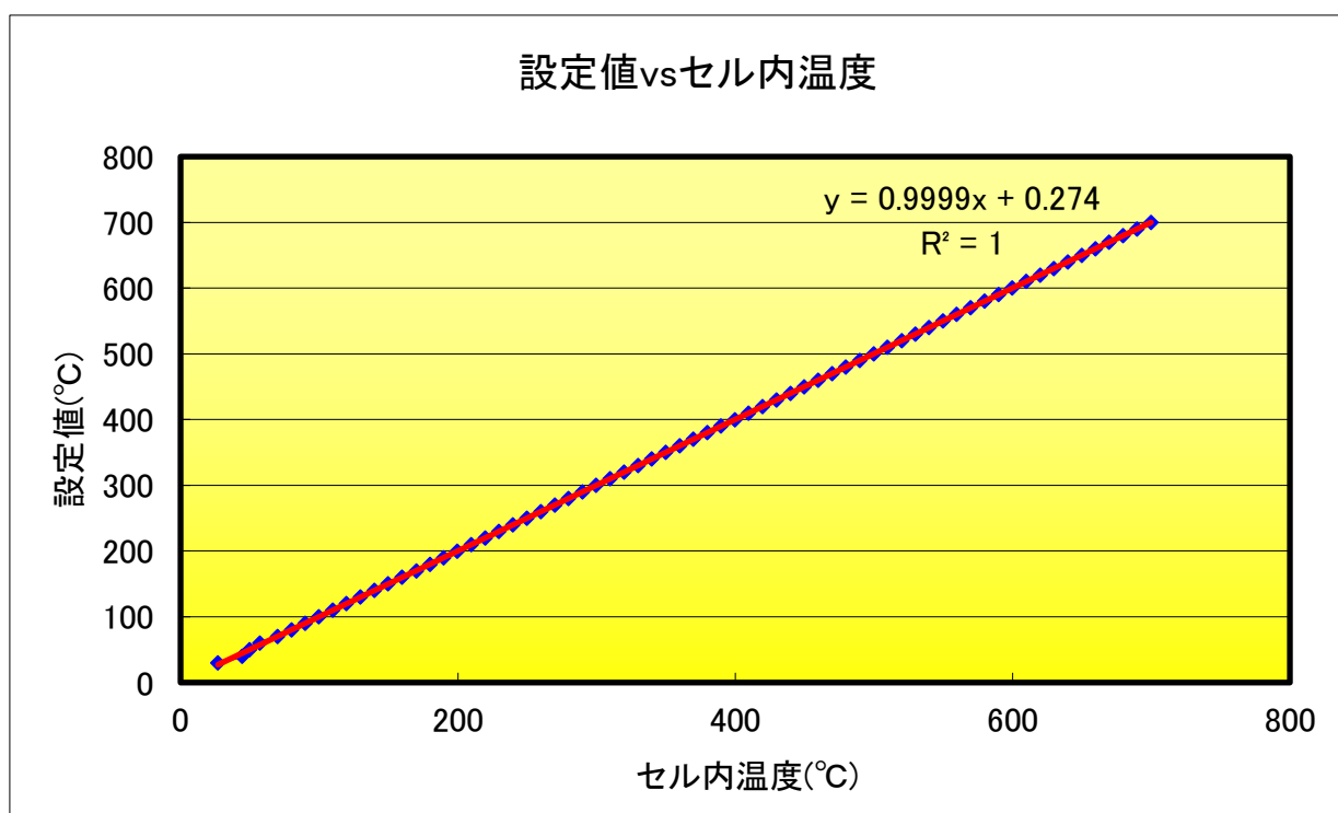
図1 設定値 vs セル内温度
