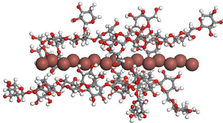
図7. キシログルカン-ヨウ素錯体モデル
