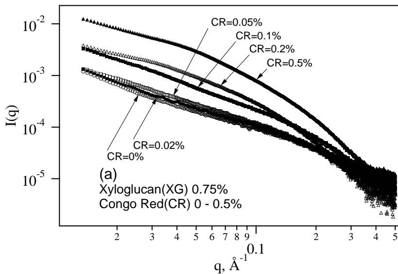
図4. コンゴレッド添加によるキシログルカングルからの小角X線散乱
