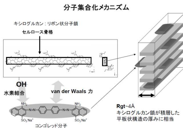
図6. キシログルカンとコンゴレッドの分子集合化メカニズム
