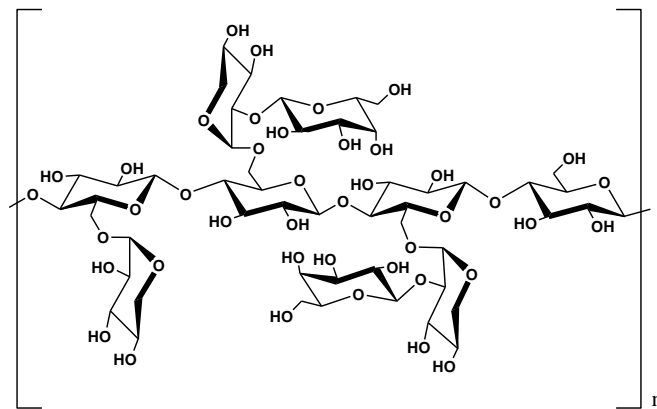
図 2. キシログルカンの化学構造.
