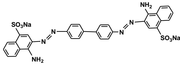
図3. コンゴレッドの化学構造
