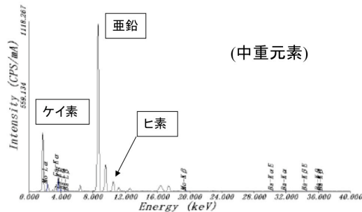
サンゴ模造品 (A1・A2)の 蛍光X線スペクトル
