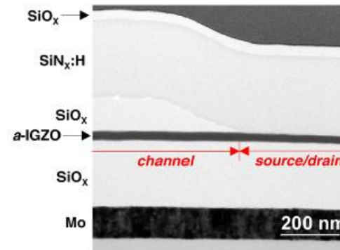
コプレーナーホモ接合TFTの提案・試作
