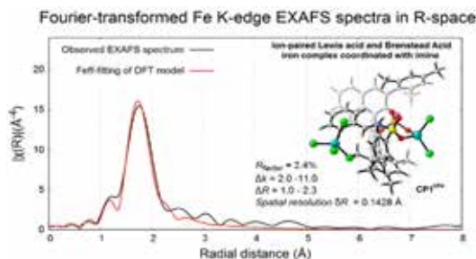
図 1. 触媒活性種の溶液構造
