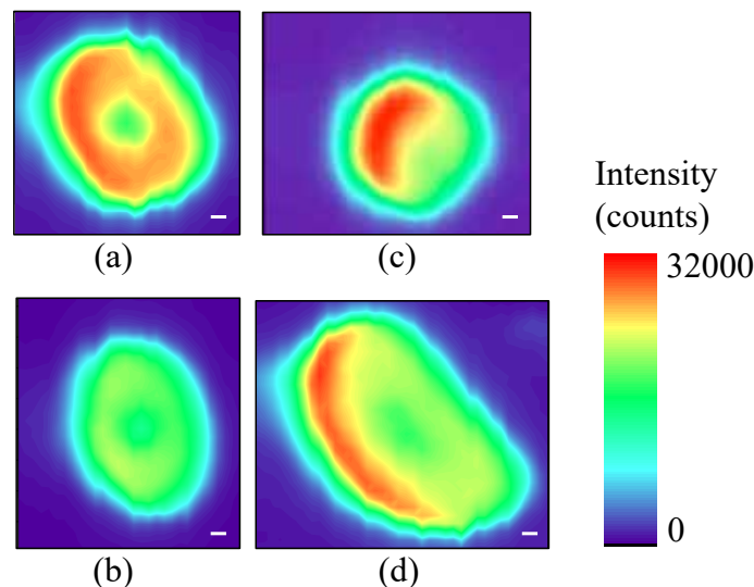
図 2. 20 代、50 代女性毛髪断面の蛍光 X 線マッピング図。(a)20 代女性毛髪、根元部、(b) 20 代女性毛髪、毛先部、(c) 50 代女性毛髪、根元部、(d) 50 代女性毛髪、毛先部。スケールバーは 10 \mu\text{m} 。
