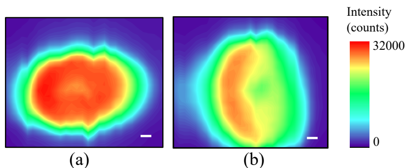
図 3. 20 代女性くせ毛髪断面の蛍光 X 線マッピング図。(a)根元部、(b)毛先部。 スケールバーは 10 \mu\text{m} 。
