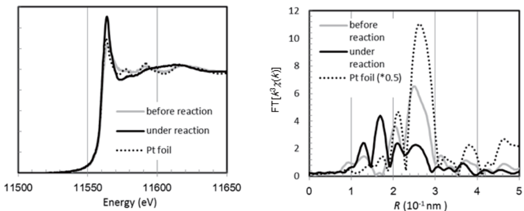
図 2. エチレン酸化反応前と反応中(室温)の Pt ナノ粒子を担持したメソポーラスシリカの Pt-L III 吸収端 XANES スペクトル(左)および動径分布関数(右)
